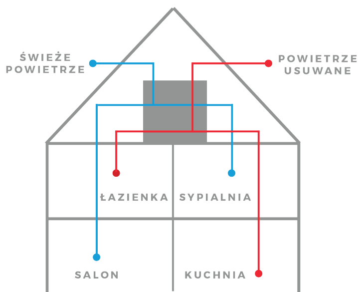
SCHEMAT DZIAŁANIA
