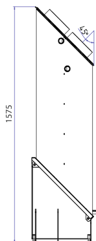
Rys 1. Wymiary wymiennika
