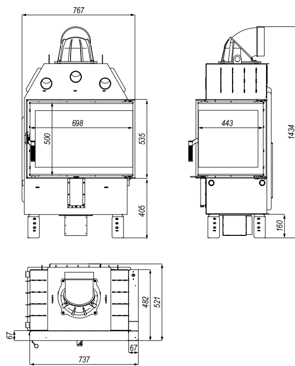
Rysunek 11. Wymiary wkładu kominkowego DEFRO HOME PRIMA SM BP.
