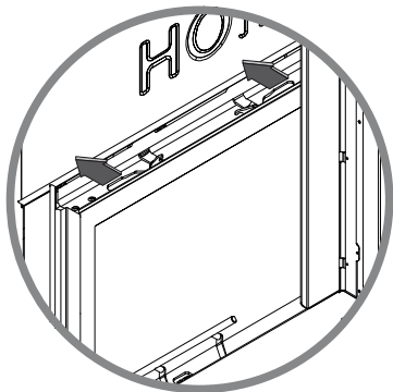
Rysunek 23. Umieszczenie rygli pozwalających na otwarcie drzwi w pozycji uchylnej w DEFRO HOME PRIMA G.
