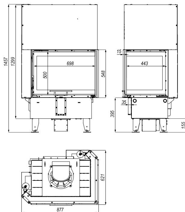
Rysunek 15. Wymiary wkładu kominkowego DEFRO HOME PRIMA SM BP G.
