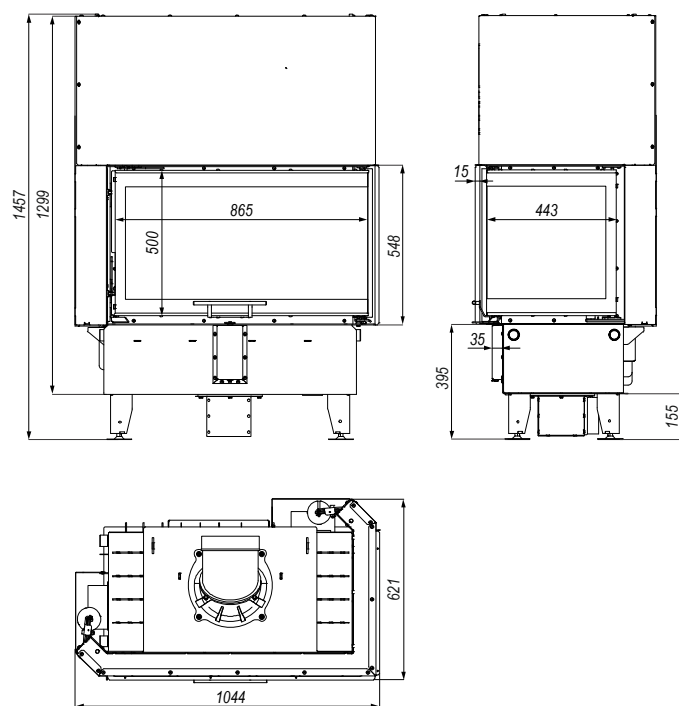
Rysunek 16. Wymiary wkładu kominkowego DEFRO HOME PRIMA ME BP G.
