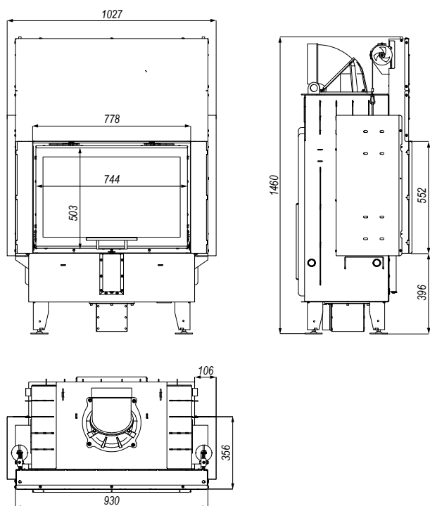
Rysunek 9. Wymiary wkładu kominkowego DEFRO HOME PRIMA ME G.
