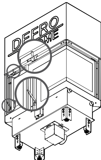
Rysunek 25. Umieszczenie rygli pozwalających na otwarcie drzwi w pozycji uchylnej w DEFRO HOME PRIMA BP G.
