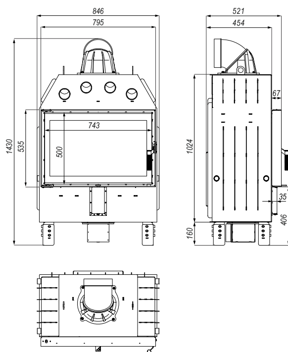
Rysunek 6. Wymiary wkładu kominkowego DEFRO HOME PRIMA ME.
