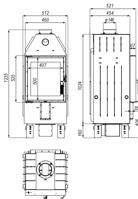
Rysunek 4. Wymiary wkładu kominkowego DEFRO HOME PRIMA XSM.
