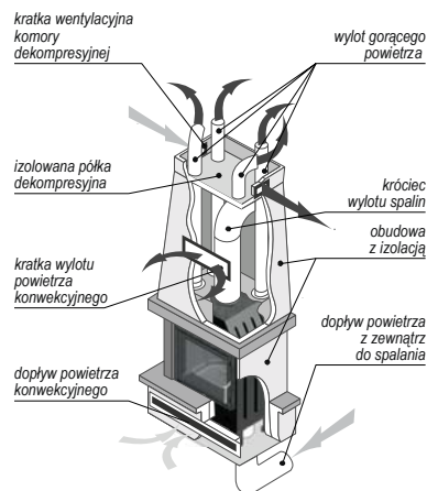
Rysunek 18. System dystrybucji gorącego powietrza.
