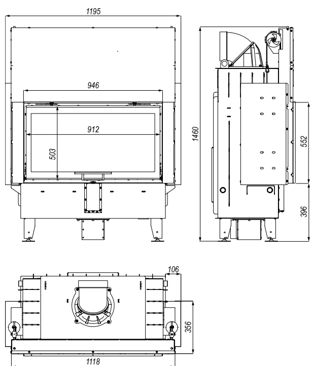
Rysunek 10. Wymiary wkładu kominkowego DEFRO HOME PRIMA LA G.
