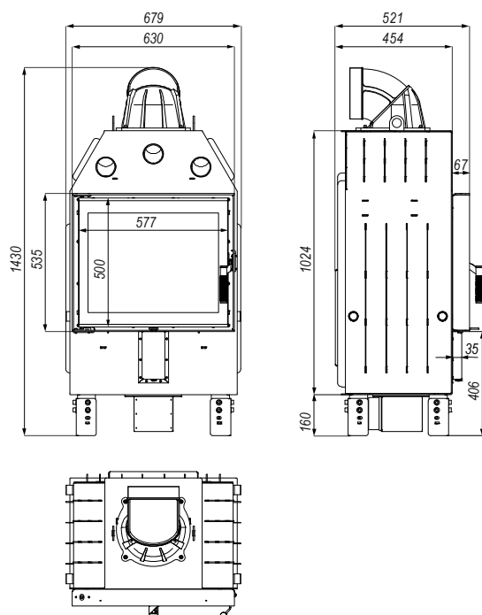
Rysunek 5. Wymiary wkładu kominkowego DEFRO HOME PRIMA SM.
