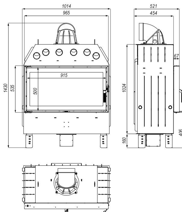
Rysunek 7. Wymiary wkładu kominkowego DEFRO HOME PRIMA LA.
