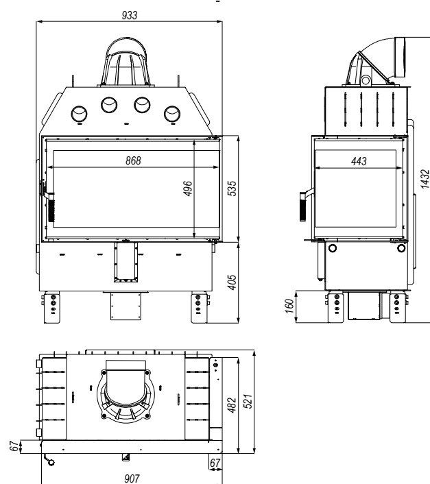
Rysunek 12. Wymiary wkładu kominkowego DEFRO HOME PRIMA ME BP.
