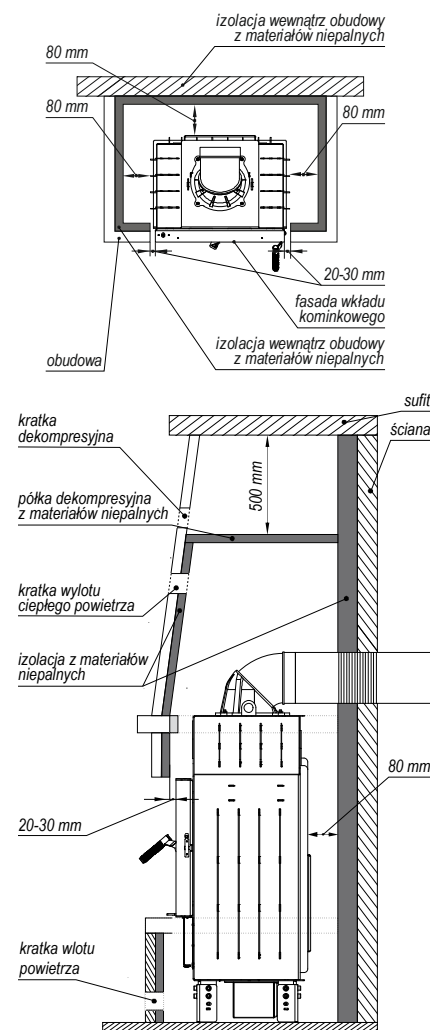
Rysunek 17. Przykładowa zabudowa wkładu kominkowego.
