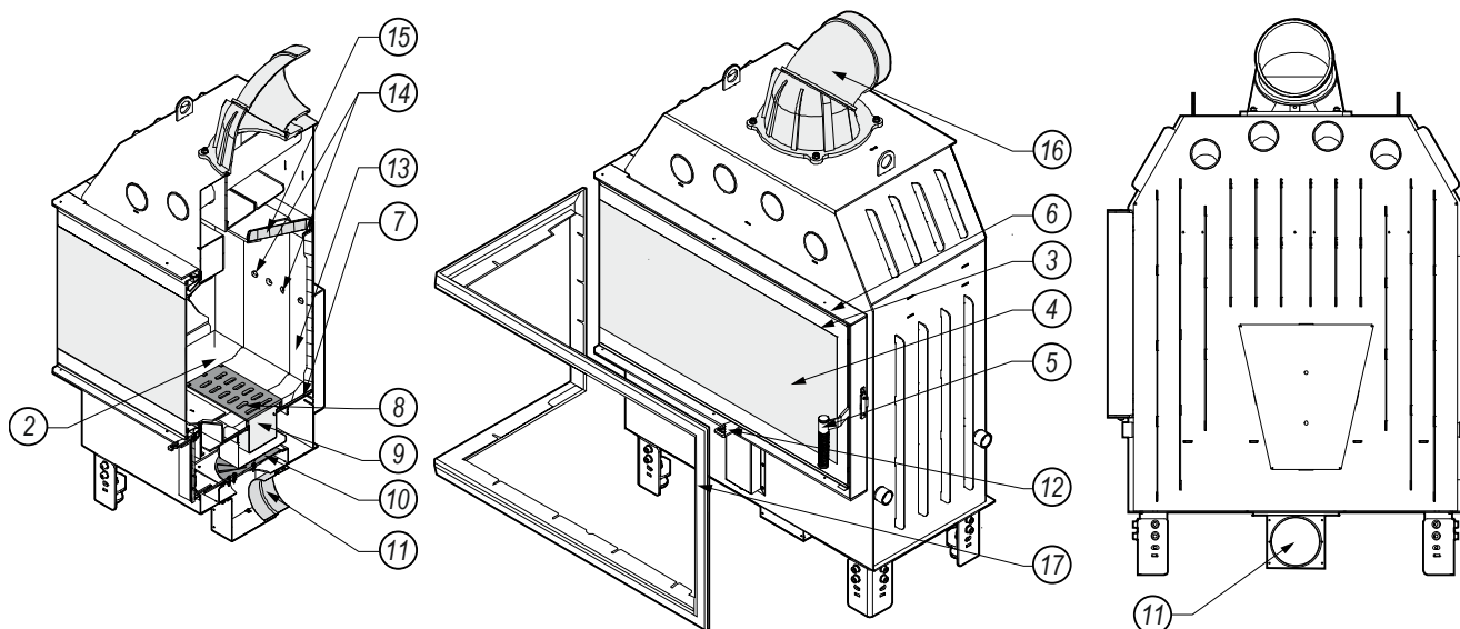
Rysunek 3. Budowa wkładu kominkowego DEFRO HOME PRIMA BL z drzwiami rozwieralnymi i szybą boczną.
