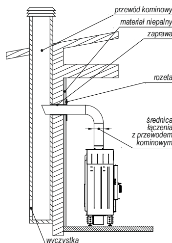
Rysunek 20. Podłączenie wkładu kominkowego do przewodu kominowego.
