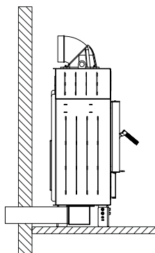
Rysunek 19. Podłączenie wkładu kominkowego do zewnętrznego wlotu powietrza.
