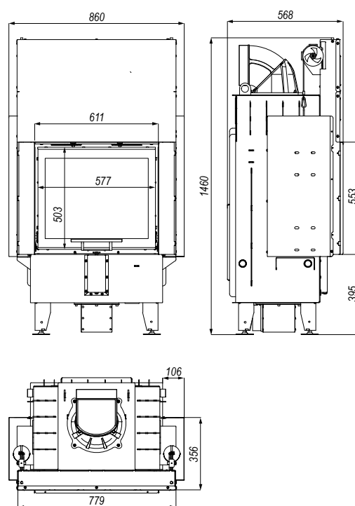
Rysunek 8. Wymiary wkładu kominkowego DEFRO HOME PRIMA SM G.
