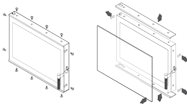
Rysunek 27. Demontaż szyby w drzwiach.
